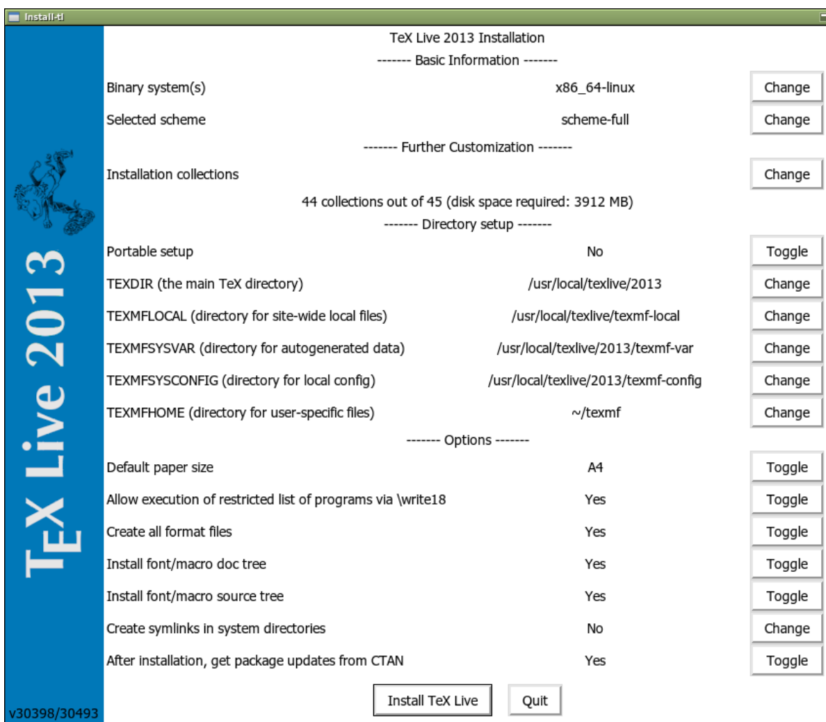
图 2: 专家模式 GUI 安装程序界面 (GNU/Linux)
