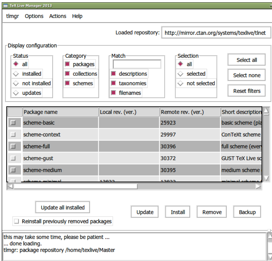
图 8: GUI 模式的 tlmgr: 按下 ‘Load’ 后的主窗口。
