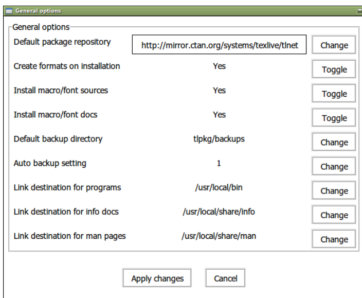
图 9: GUI 模式的 tlmgr: 通用选项
